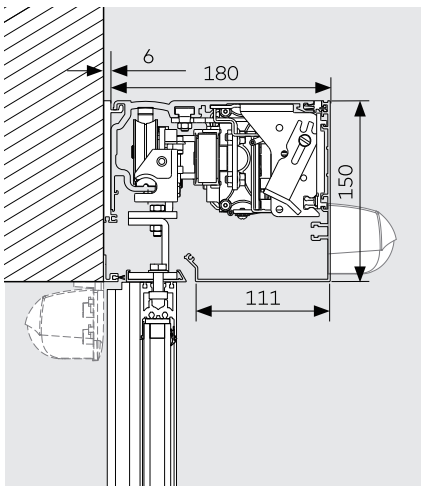
墙面安装示意图： 机组高度 150mm
